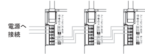
送り配線の例
